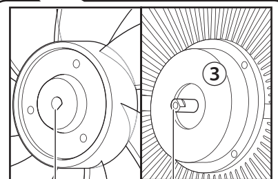
羽根をモーター軸の形状に合わせてはめ込む
