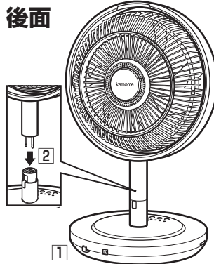
低くする場合 高さ約57.0cm
