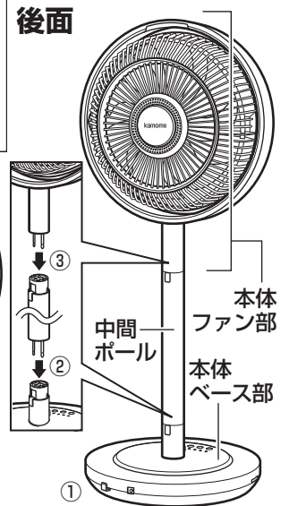
高くする場合 高さ約83.0cm
