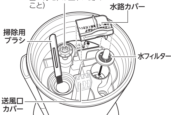
水路カバー
