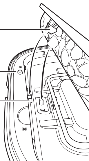
固定フック
